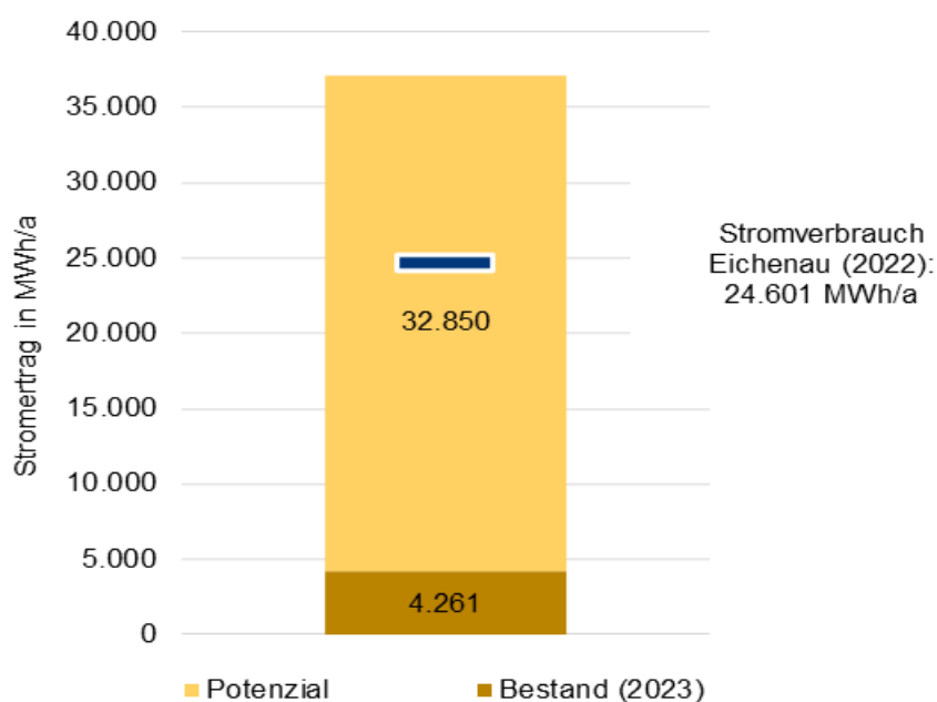
Abbildung 22: Ausbaupotenzial für Dach-Photovoltaikanlagen.
