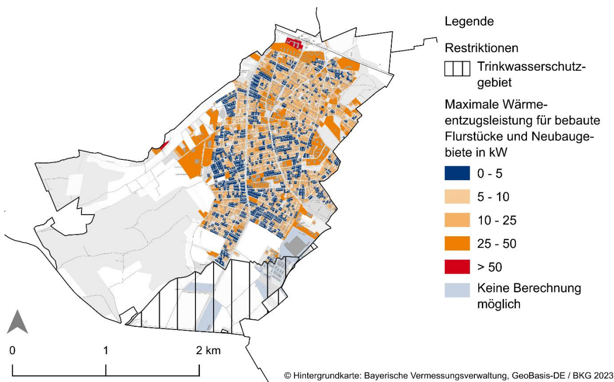
Abbildung 30: Potenzialkarte für Erdwärmekollektoren.
