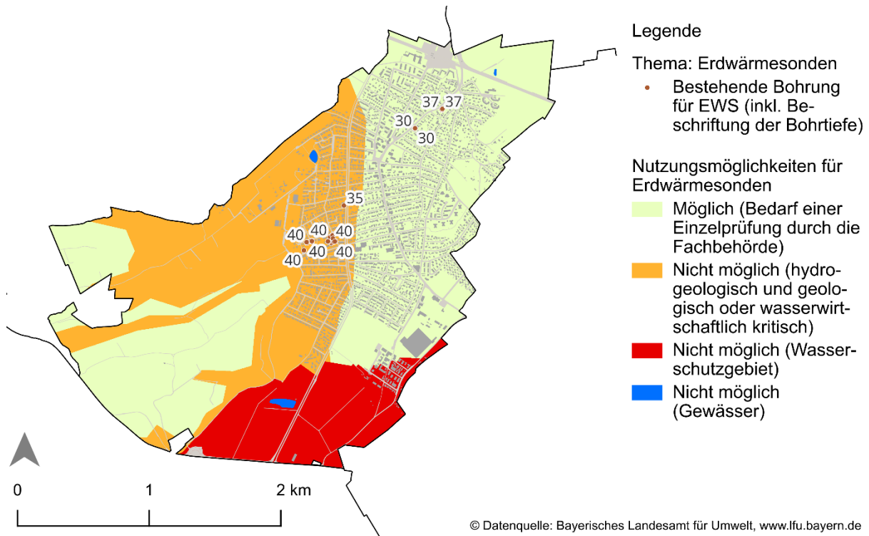
Abbildung 34: Potenzialkarte für Erdwärmesonden.
