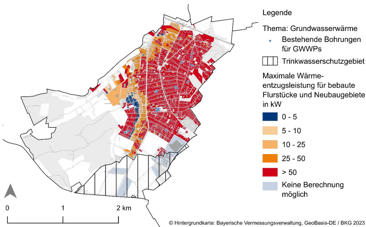
Abbildung 32: Potenzialkarte für Grundwasserwärmepumpen.
