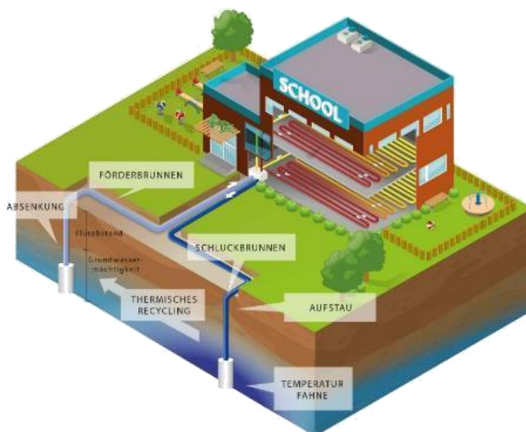
Abbildung 31: Typischer Aufbau einer Grundwasserwärmepumpe mit Förder- und Schluckbrunnen (Bildquelle: Interreg Alpine Space Programme, Projekt GRETA).
