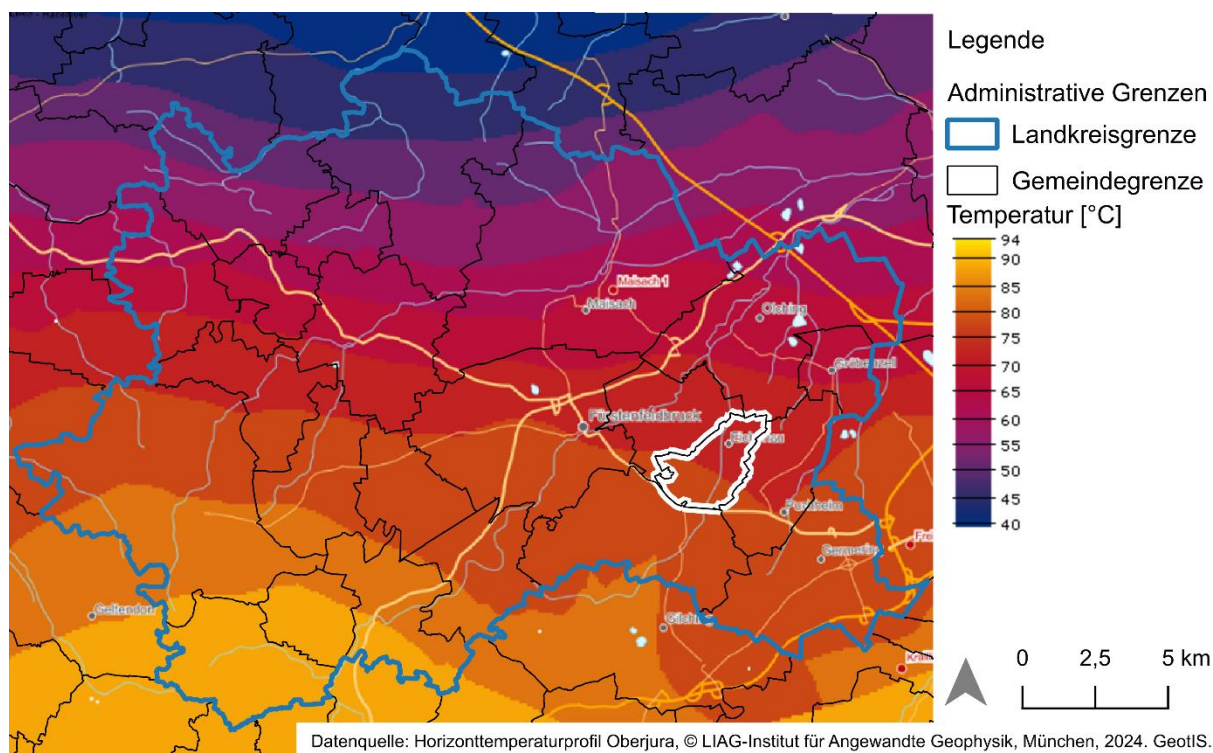
Abbildung 35: Horizonttemperatur entlang des Oberjuras (Datenquelle: GeotIS).
