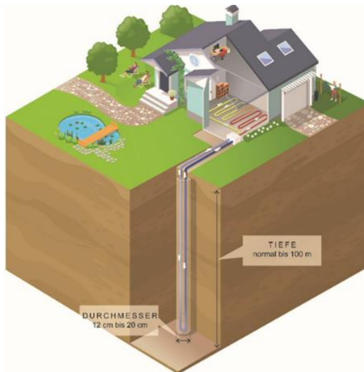
Abbildung 33: Typischer Aufbau einer Erdwärmesonde (Bildquelle: Interreg Alpine Space Programme, Projekt GRETA).
