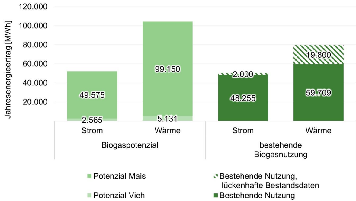
Abbildung 27: Summiertes Potenzial zur Energieerzeugung aus Biogas im Landkreis.
